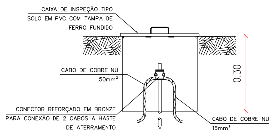
1 DET. - CAIXA DE INSPEÇÃO SEM ESCALA
