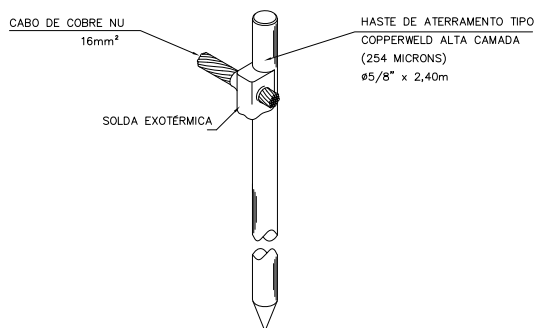
2 DET. - HASTE DE ATERRAMENTO SEM ESCALA
